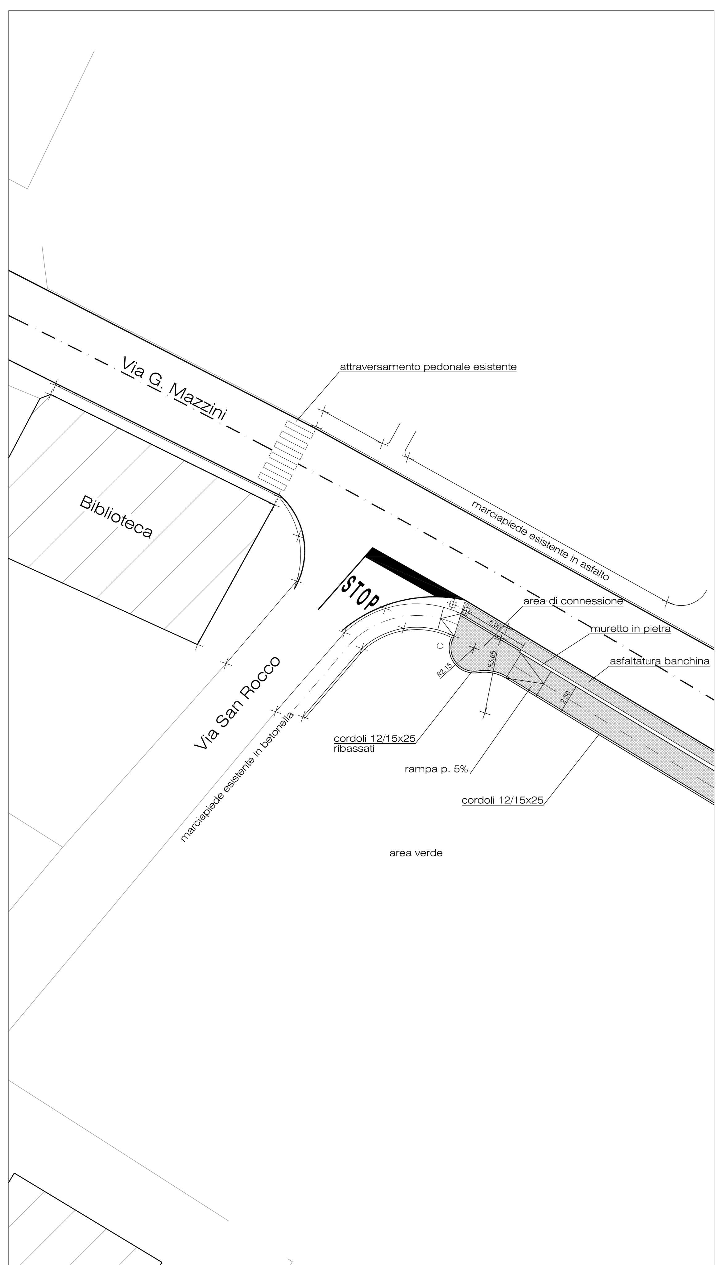
DETTAGLIO -1-
