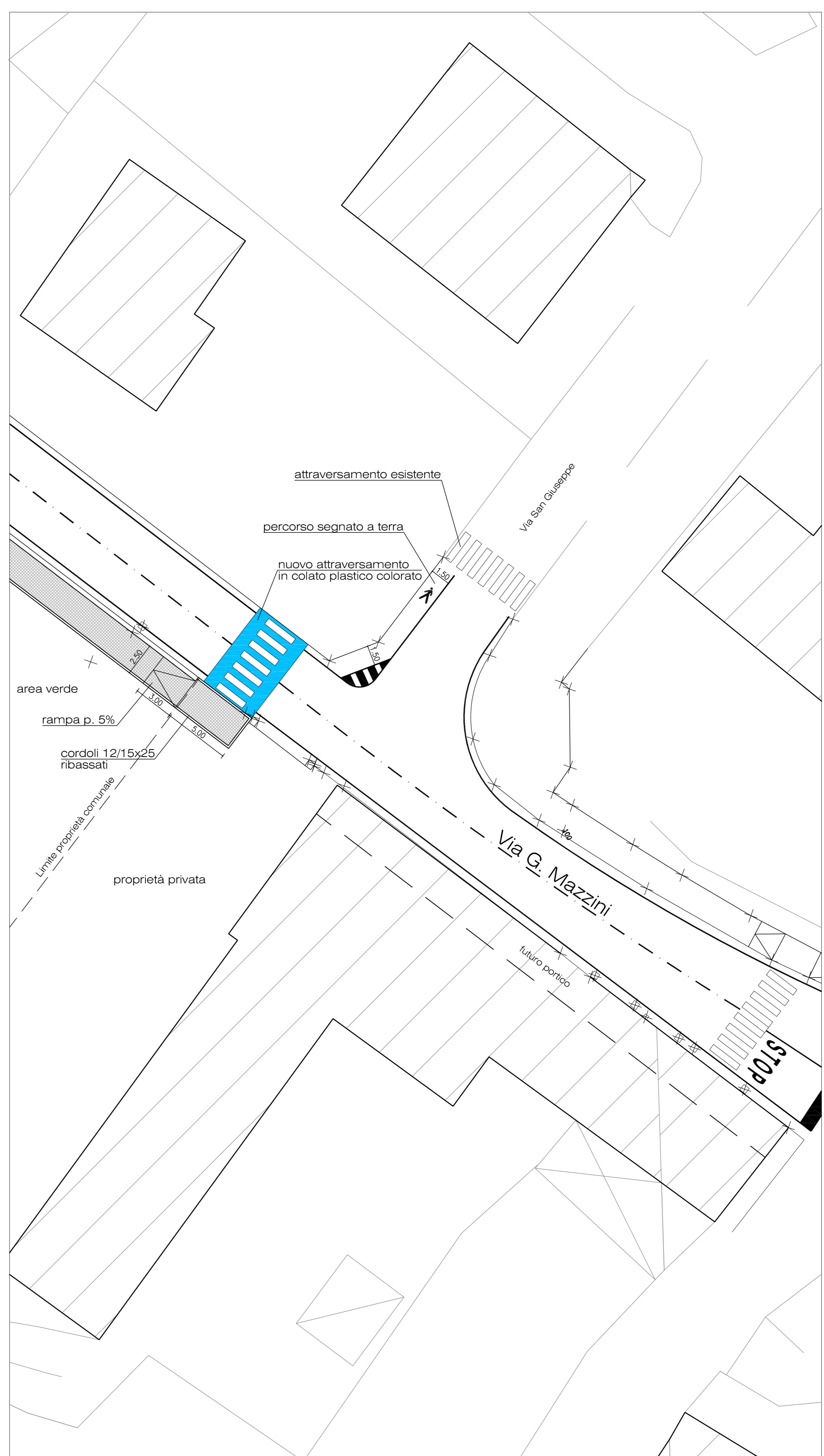
DETTAGLIO -3-
